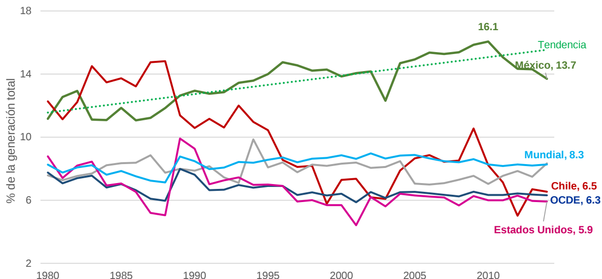
Gráfica 1. Pérdidas de electricidad en transmisión y distribución
