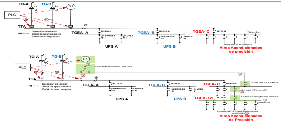
Figura 1 Instalación actual e instalación futura
