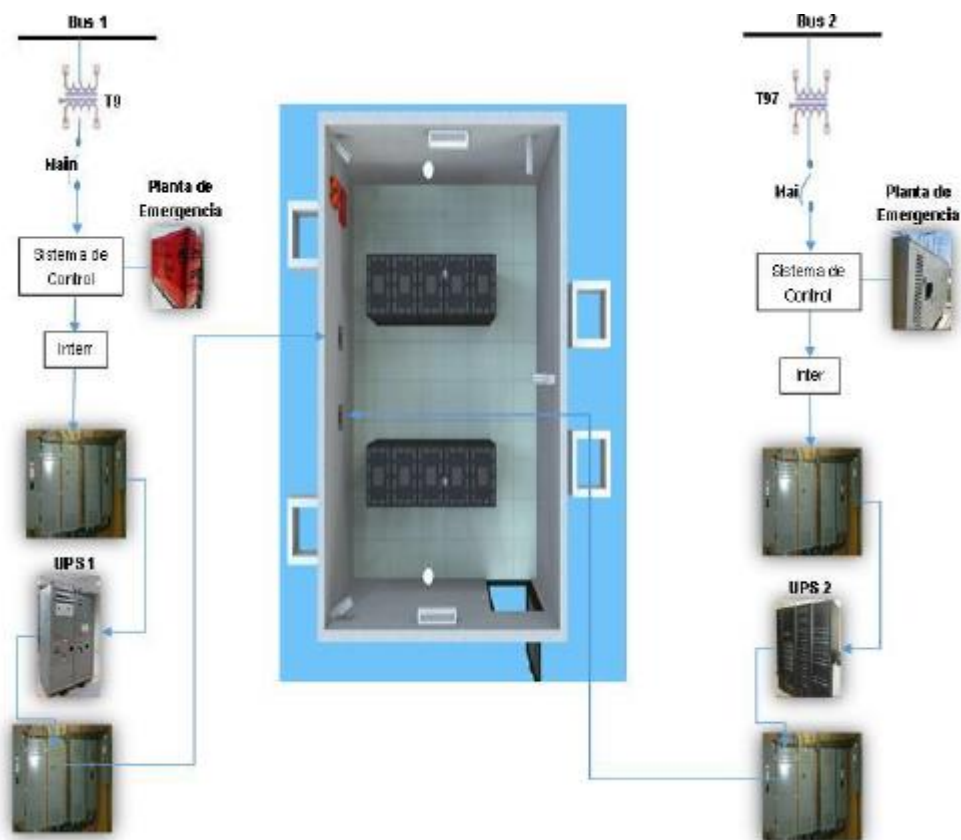
Figura 1 Diagrama eléctrico
