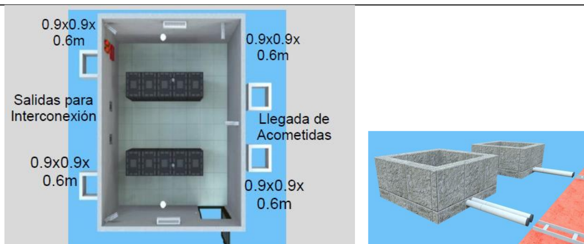
Fig 4.5 Detalle de registros
