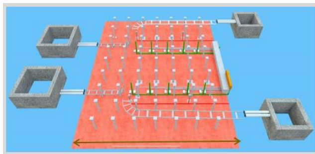
Fig. 14 Canalizaciones en piso falso
