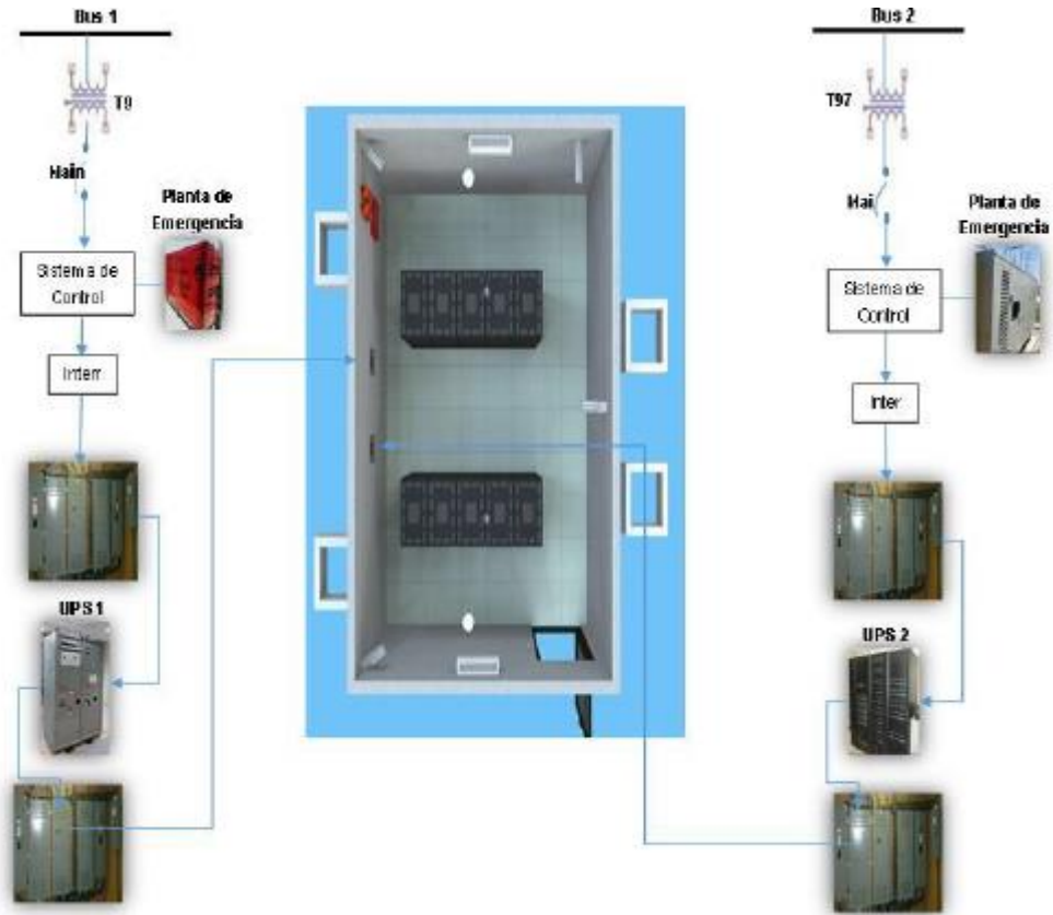
Figura 1 Diagrama eléctrico
