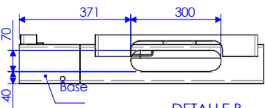
DETALLE B ESCALA 2 : 35 Entrada de cables.
