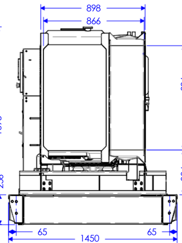
VISTA LATERAL
