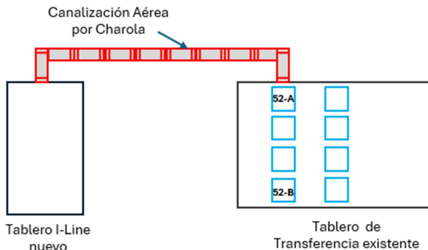
Diagrama 1. Canalización de instalación, Partida 1.
